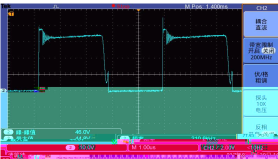
11. 18V MOS
